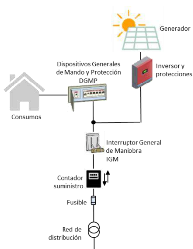
Figura 11: Conexión a la Derivación Individual (DI). P < 800 \text{ VA}
