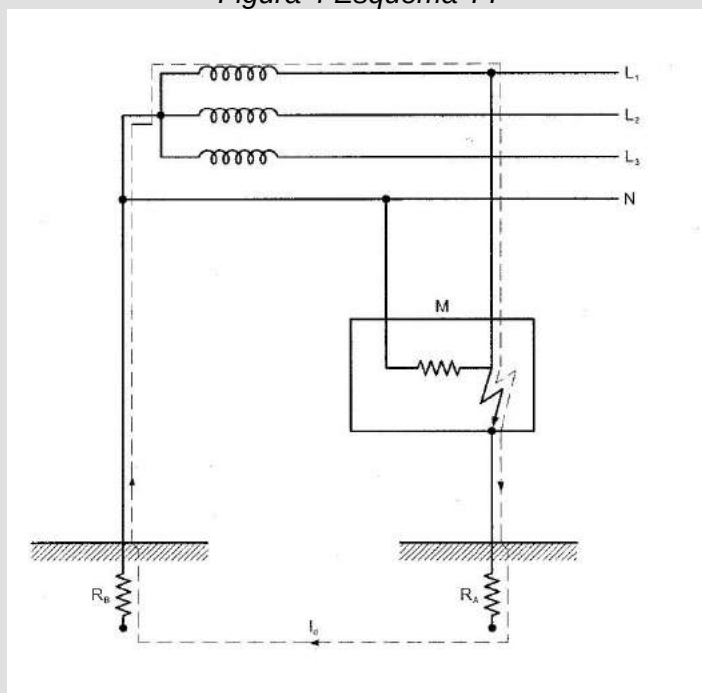
Figura 4 Esquema TT
